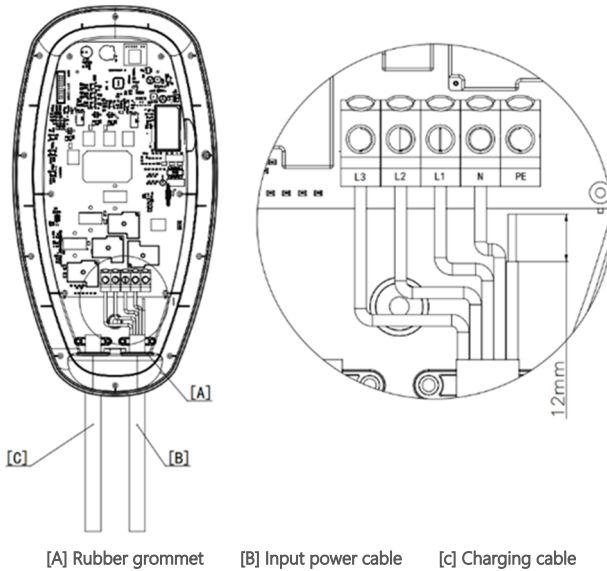
Fig. 5-9 Wiring
