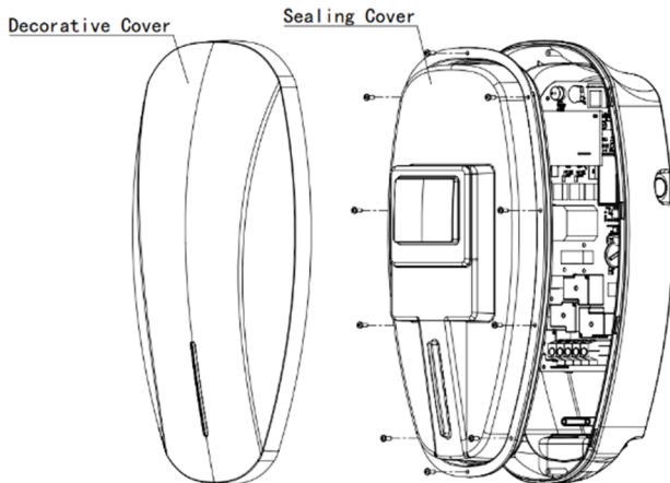
Fig. 5-10 Close the lid
