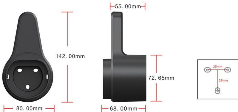
Fig. 5-9 Empty socket
